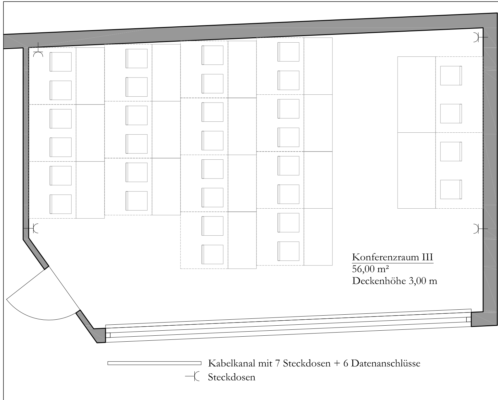
Fleming's Hotel München Schwabing Grundriss Konferenzraum III Maßstab 1:50
