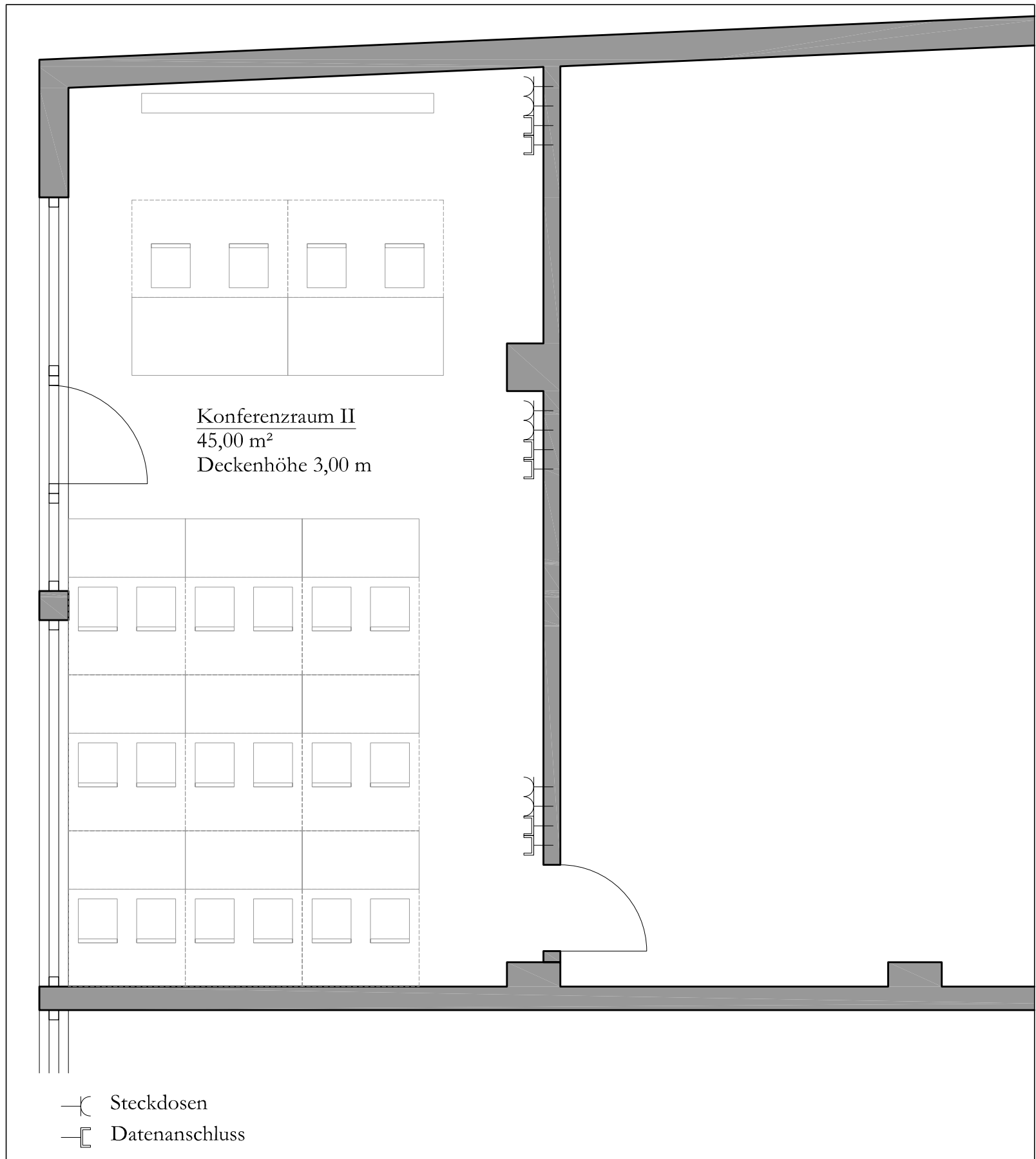
Fleming's Hotel München Schwabing Grundriss Konferenzraum II Maßstab 1:50
